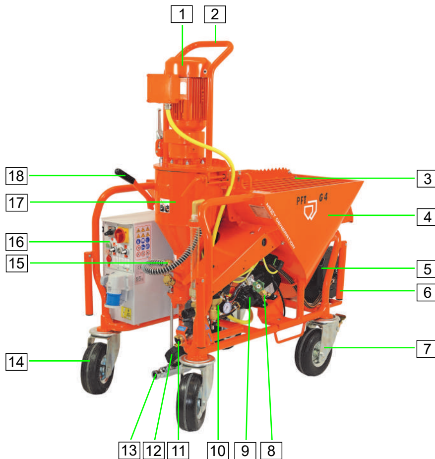
Abb. 8: Übersicht über die Baugruppen
