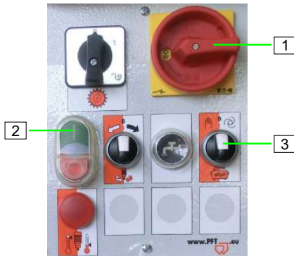
Abb. 41: Maschine einschalten
