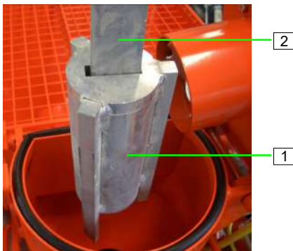
Abb. 82: Mischrohrreiniger einsetzen
