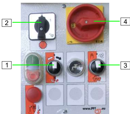
Abb. 87: Rückwärtslauf
