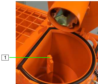
Abb. 81: Motorkippflansch öffnen
