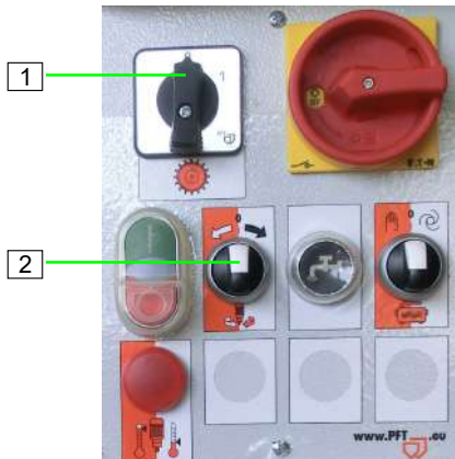
Abb. 76: Arbeitsende
