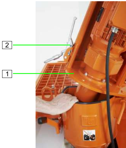
Abb. 83: Motorkippflansch schließen
