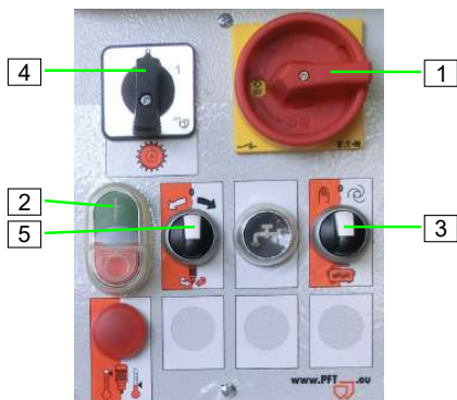
Abb. 58: Maschine einschalten
