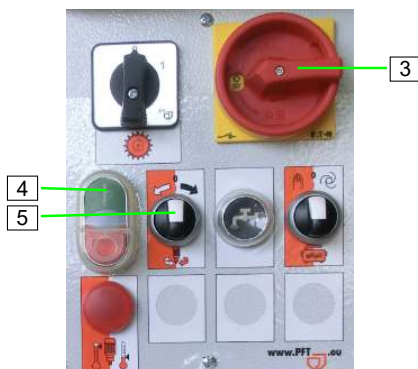
Abb. 84: Mischrohr reinigen
