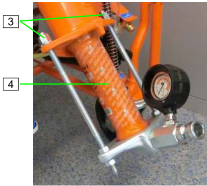
Abb. 98: Pumpe wechseln
