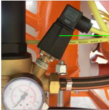
Abb. 95: Druckschalter Wasser
