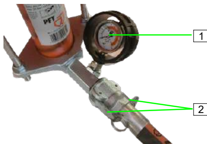
Abb. 77: Mörtelschlauch abkuppeln
