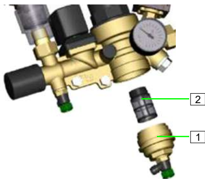
Abb. 94: Schmutzfängersieb
