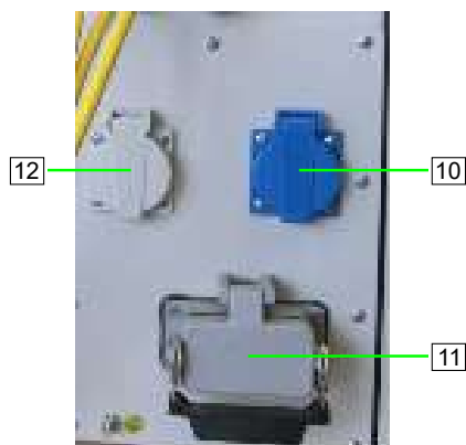
Abb. 12: Baugruppe Schaltschrank
