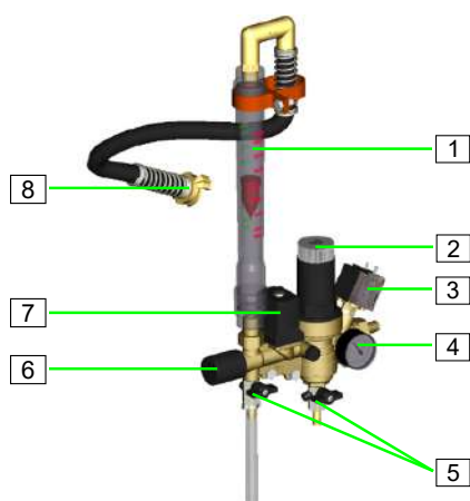
Abb. 15: Baugruppe Wasserarmatur
