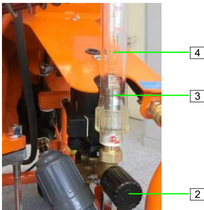
Abb. 43: Wassermenge einstellen
