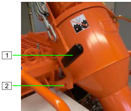
Abb. 97: Mischrohr hochklappen
