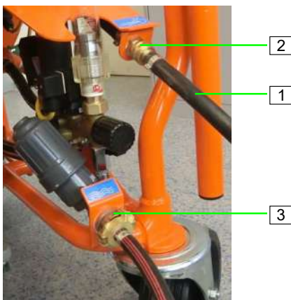
Abb. 73: Wasserarmatur trocknen
