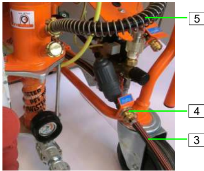
Abb. 38: Wasser anschließen
