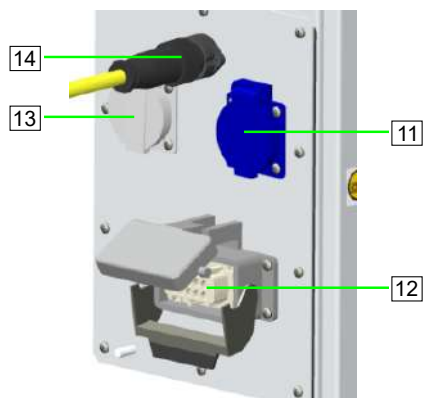
Abb. 13: Baugruppe Schaltschrank
